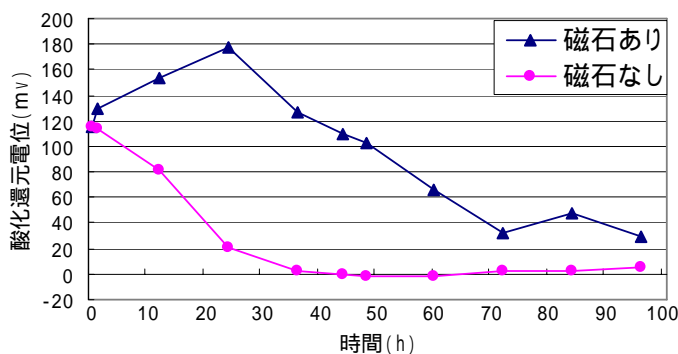
図-6 酸化還元電位
