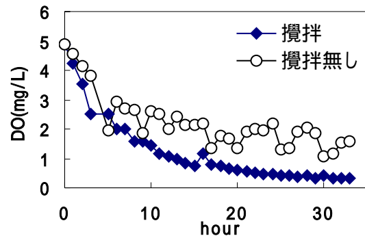
図 - 6 DO 変化
