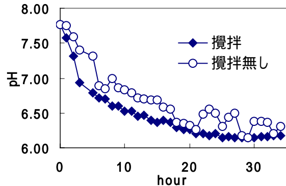
図 - 5 pH 変化
