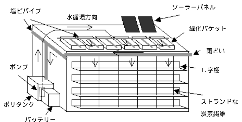
図1 構造物緑化の構想図
