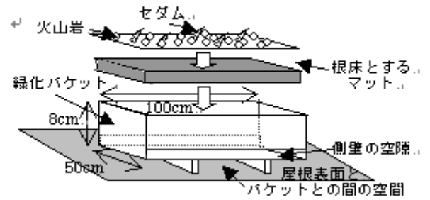
図2 緑化バケットの構造図
